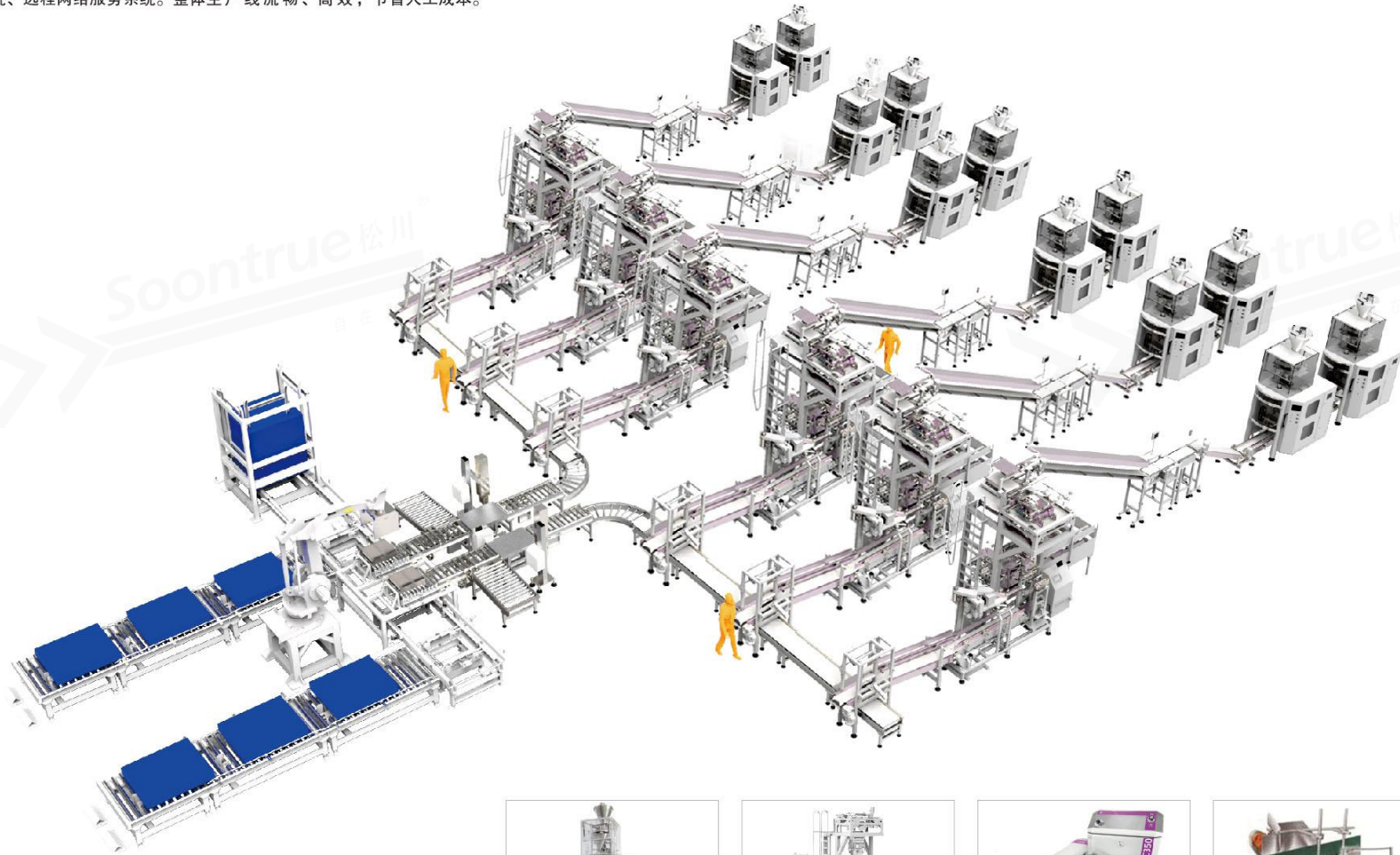
枕形背封包装系统
